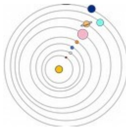
système solaire
