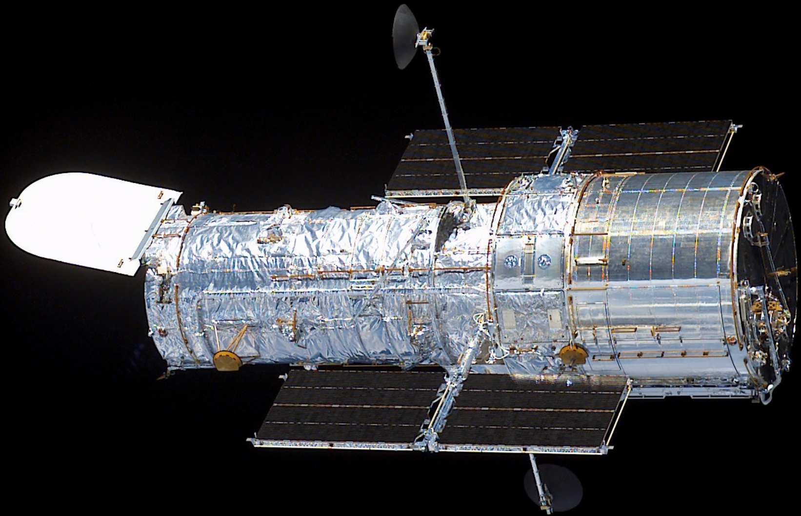
Télescope Hubble
